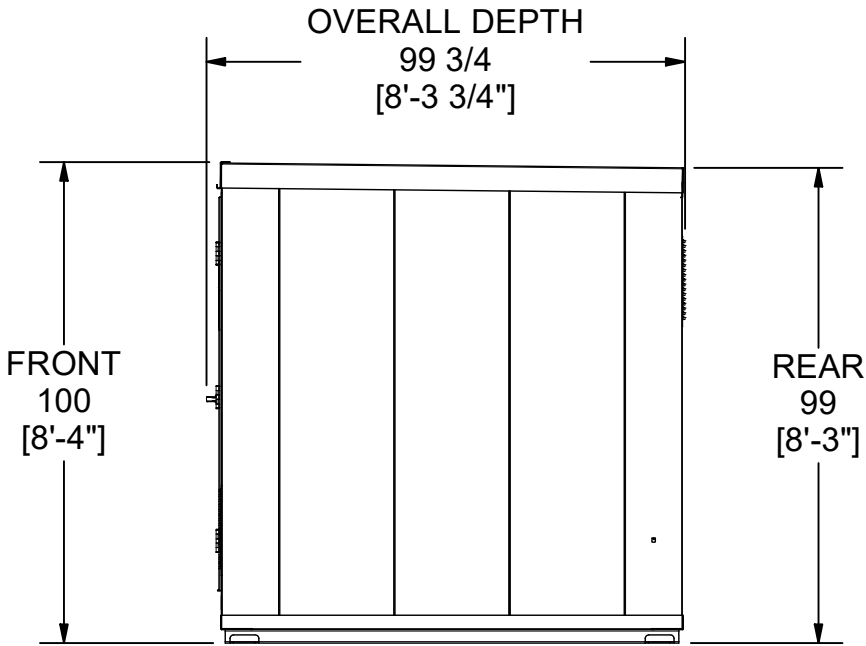
RIGHT ELEVATION
